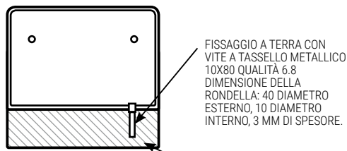
SEZIONE D-D
