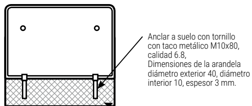
SECCIÓN D-D
